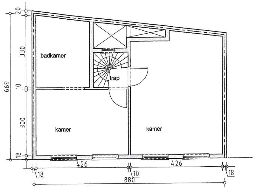
niveau +2 (bestaande toestand)
