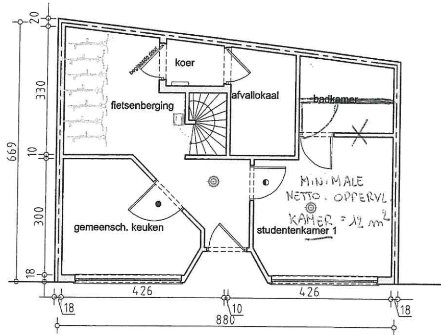
niveau 00 (nieuwe toestand)
