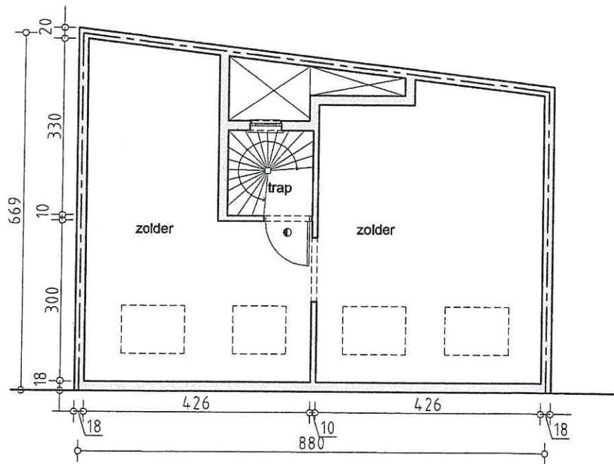
niveau +3 (bestaande toestand)
