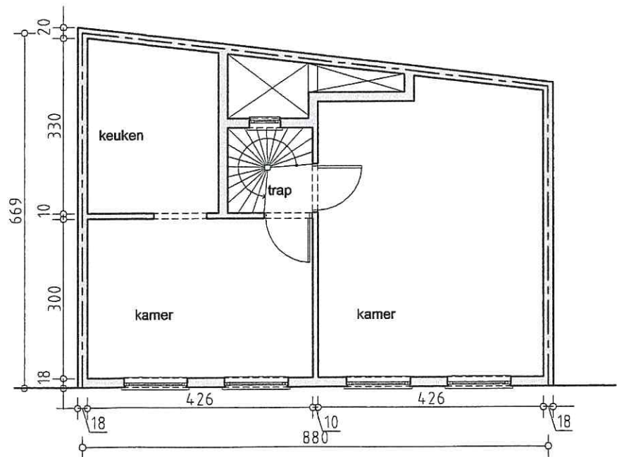
niveau +1 (bestaande toestand)
