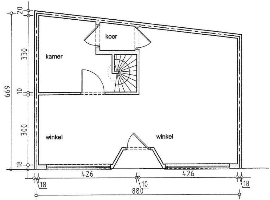
niveau 00 (bestaande toestand)
