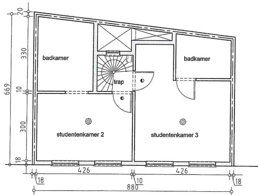
niveau +1 (nieuwe toestand)
